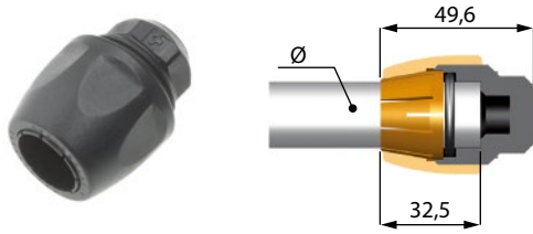
不锈钢管堵
